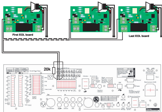
Подключение нескольких плат к одному входу управления
