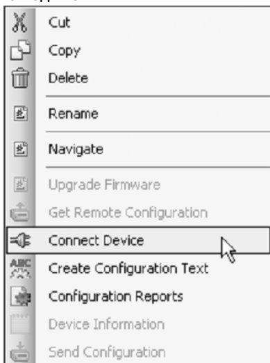
Рисунок 4. ОКНО ПОДКЛЮЧЕНИЯ
