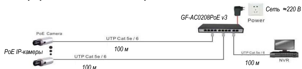
Рис. 1 Схема подключения сетевых устройств
