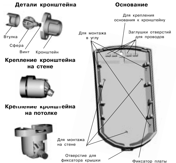
Рис. 2. Основание извещателя и кронштейн
