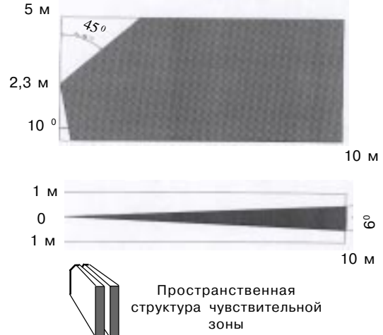
Рис. 1. Диаграмма зоны обнаружения
