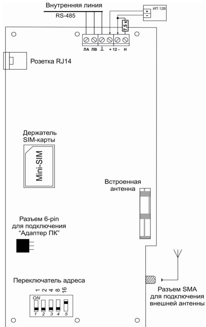
Рис 2. Схема внешних соединений блока автодозвона
