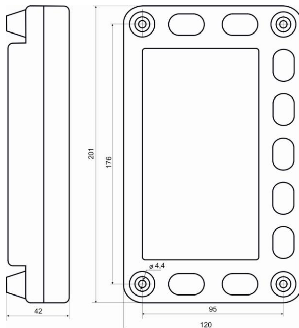
Рис 3. Габаритные и установочные размеры блока автодозвона
