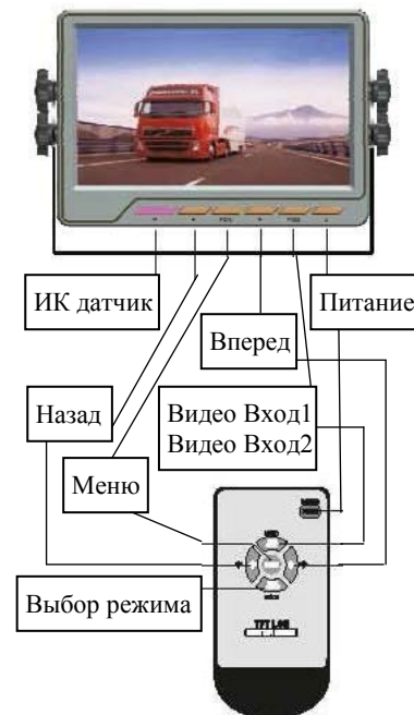
Рис. 3 Органы управления
