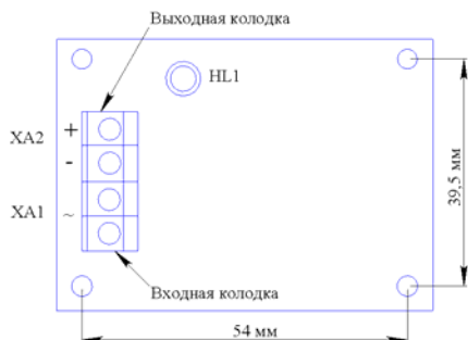
Рисунок – Преобразователь напряжения ПН-24АС/12-1,0
