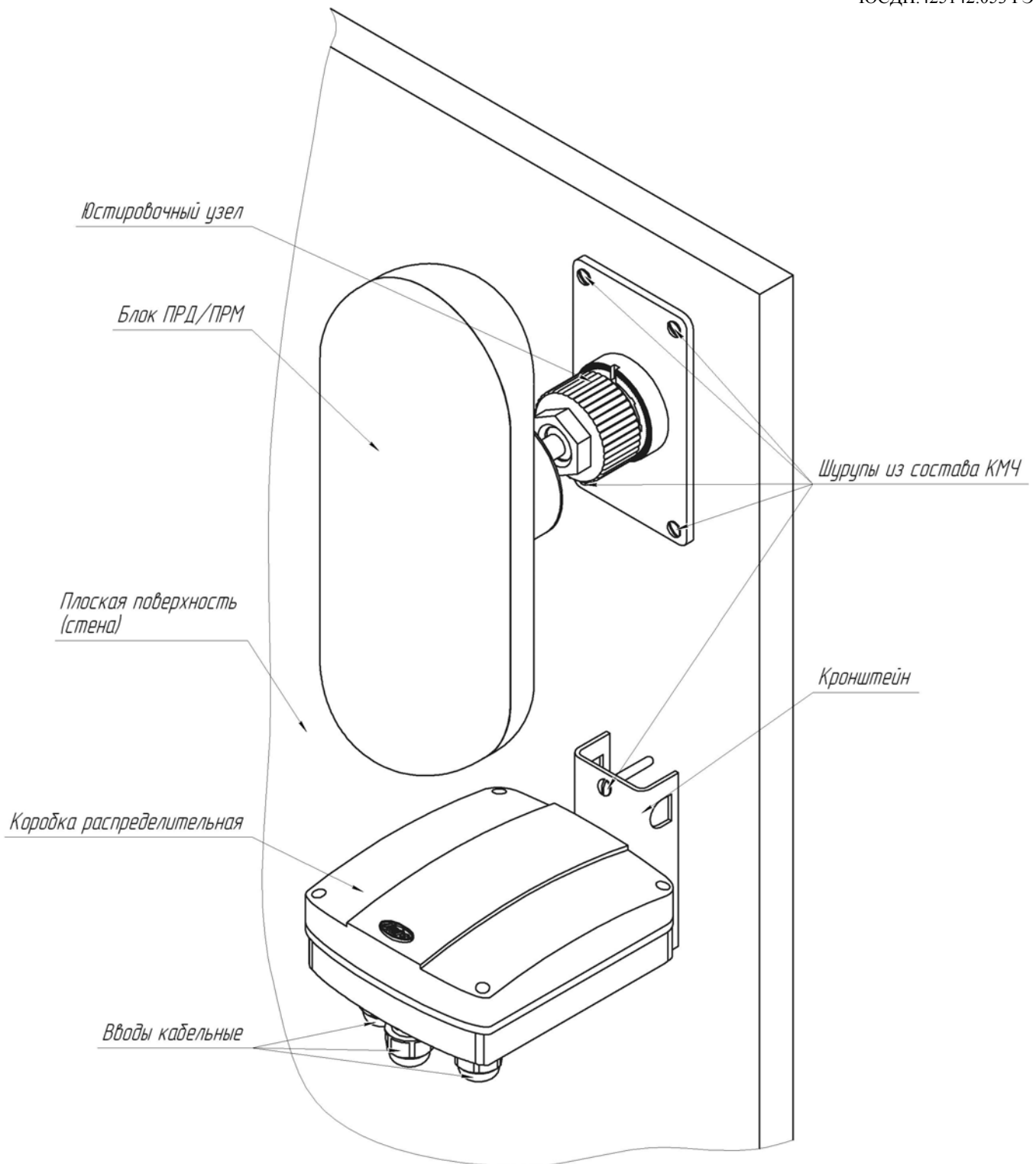
Рисунок 1.3 – Внешний вид блоков ПРМ /ПРД «ТАНТАЛ-600-01» и КР на плоской поверхности (стене)
