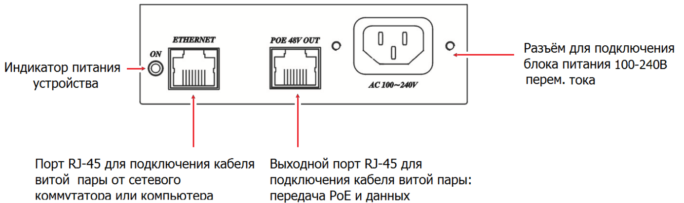
Рис.3 Разъёмы инжектора IP05I.
