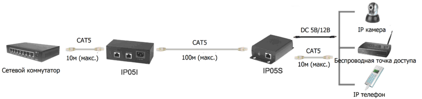
Рис.2 Схема подключения инжектора IP05I и сплиттера IP05S.
