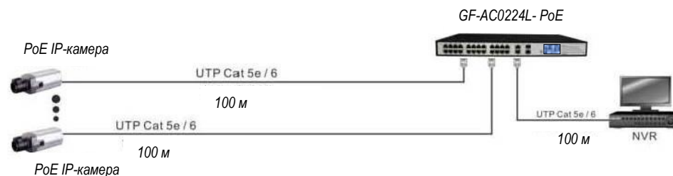
Рис. 1 Схема подключения сетевых устройств
