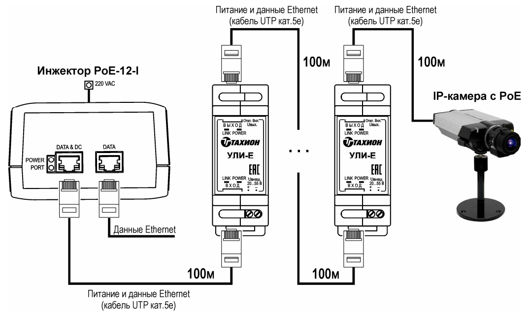
Рис.4 Пример удлинения линии связи с двумя и более УЛИ-Е
