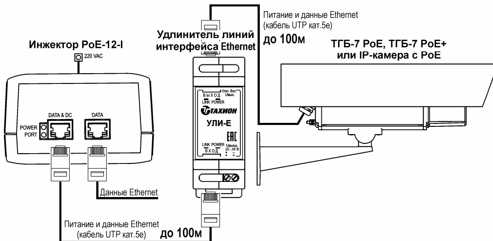
Рис.3 Пример удлинения линии связи с УЛИ-Е
