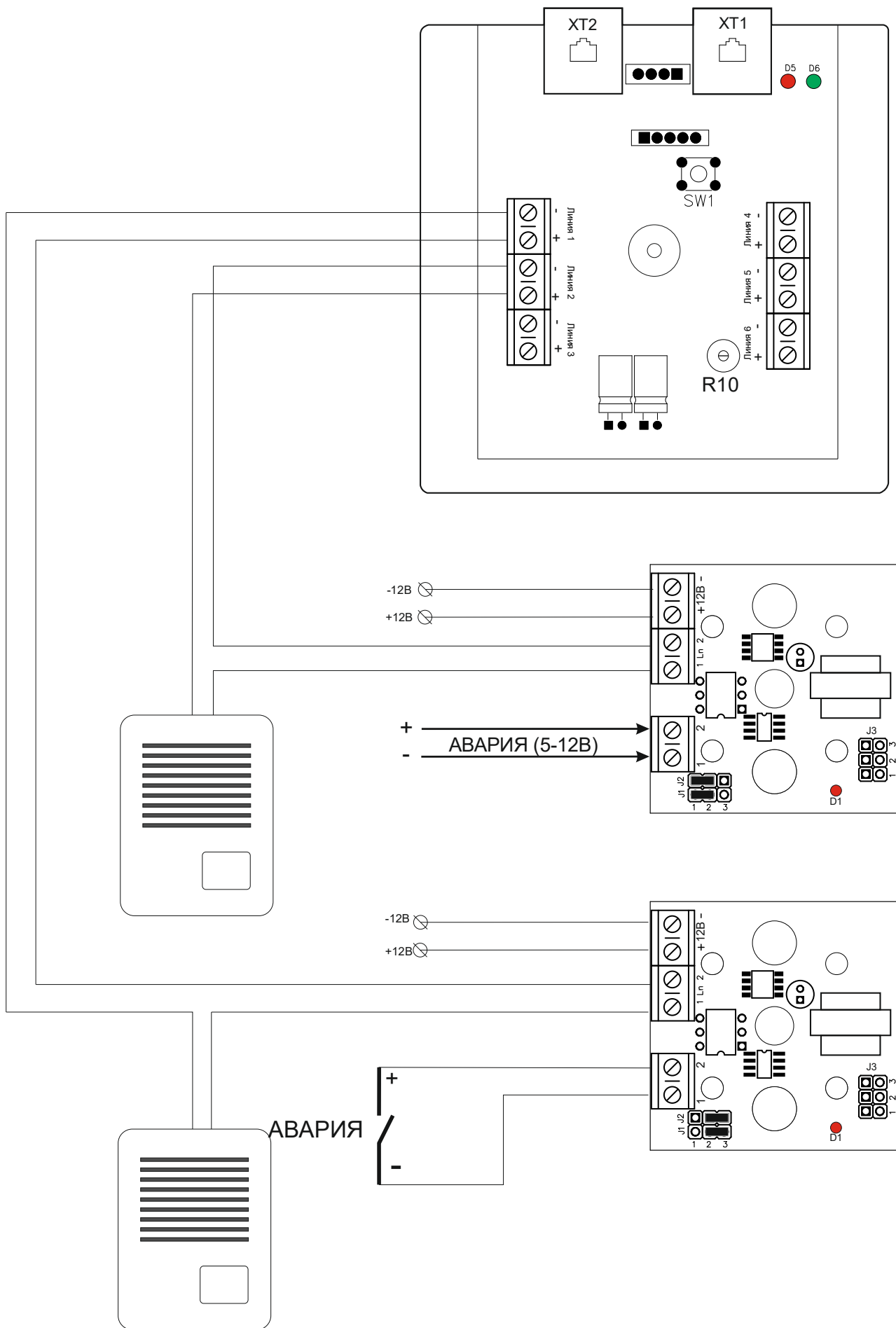
Рисунок 3. Схема подключения
