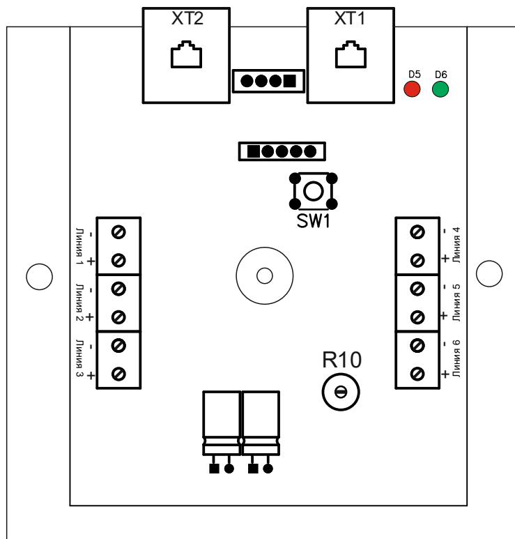
Рисунок 1. Внешний вид приемника GC-3006R1
