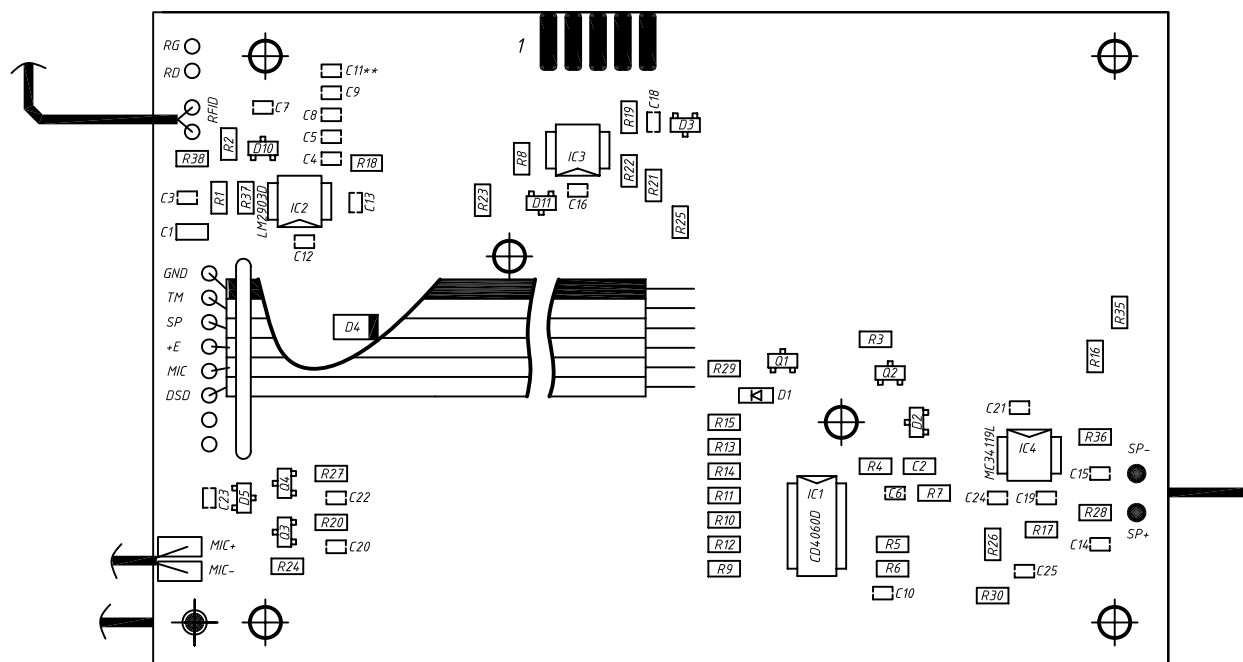
Плата БВД-313R Сборочный чертеж
