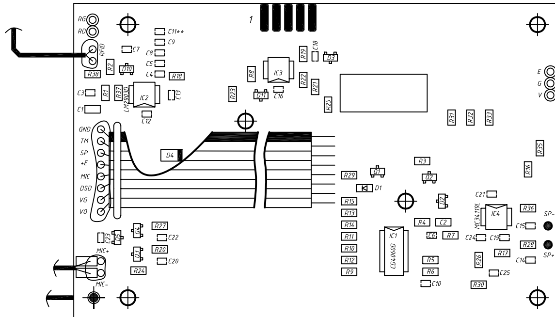
Плата БВД-313RCP Сборочный чертеж
