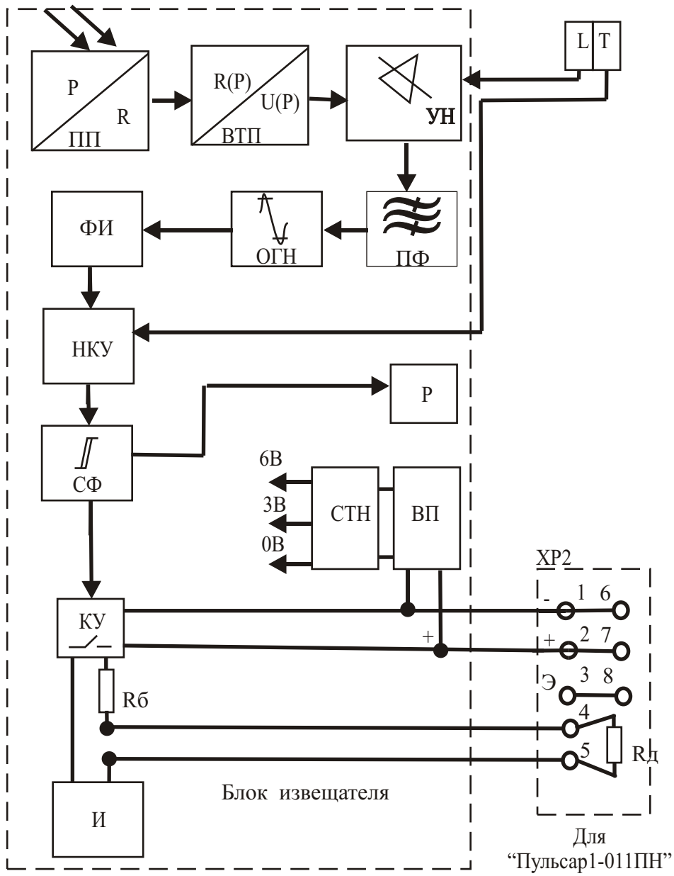
Рис 3 Схема функциональная
