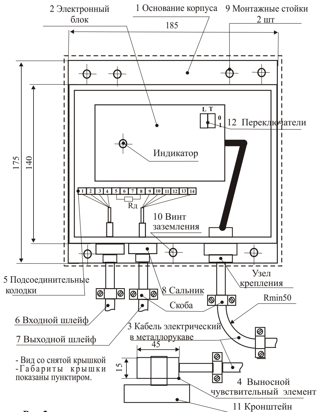
Рис 2 Извещатель "Пulsar1-011П"
