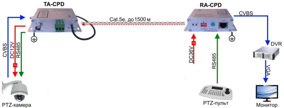
Рис.4 Схема подключения передатчика TA-CPD и приемника RA-CPD
