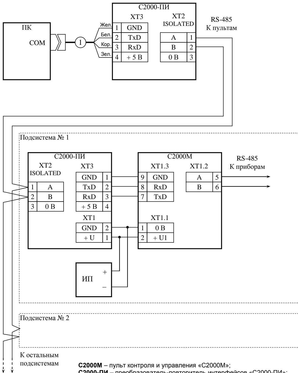
Рисунок 9 Схема подключения нескольких пультов «С2000М» к персональному компьютеру с АРМ «Орион» с гальванической изоляцией интерфейса RS-485
