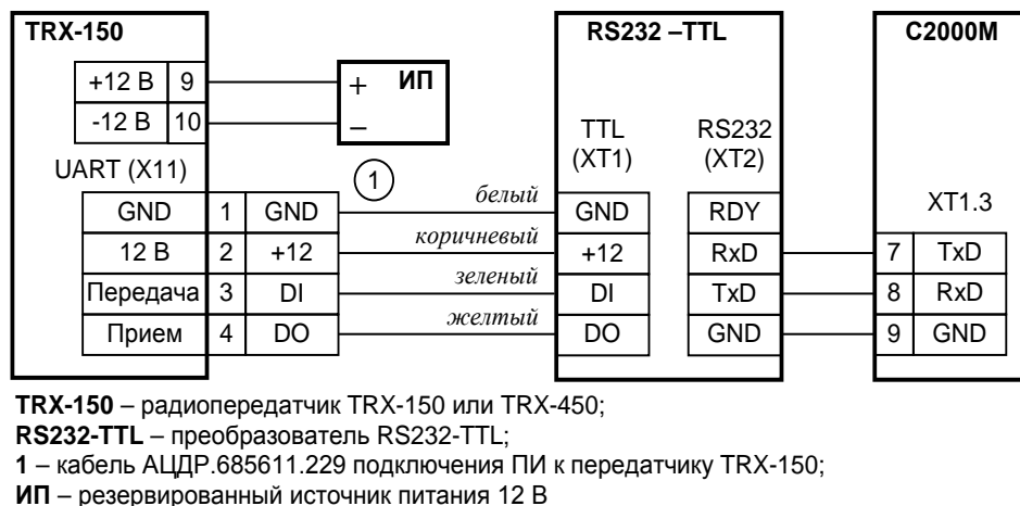
Рисунок 13 Схема подключения радиопередатчика TRX-150 к пульту «С2000М»
