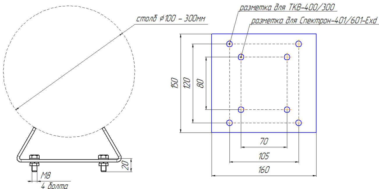
Рис. 1 – Габаритные размеры
