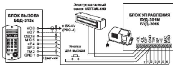
Рисунок 3 - Схема соединений блока вызова БВД-313х с блоком управления БУД-301М, БУД-301К, электромагнитным замком VIZIT-ML400 и кнопкой для выхода
