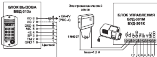
Рисунок 4 - Схема соединений блока вызова БВД-313х с блоком управления БУД-301М, БУД-301К и электромагнитным замком
